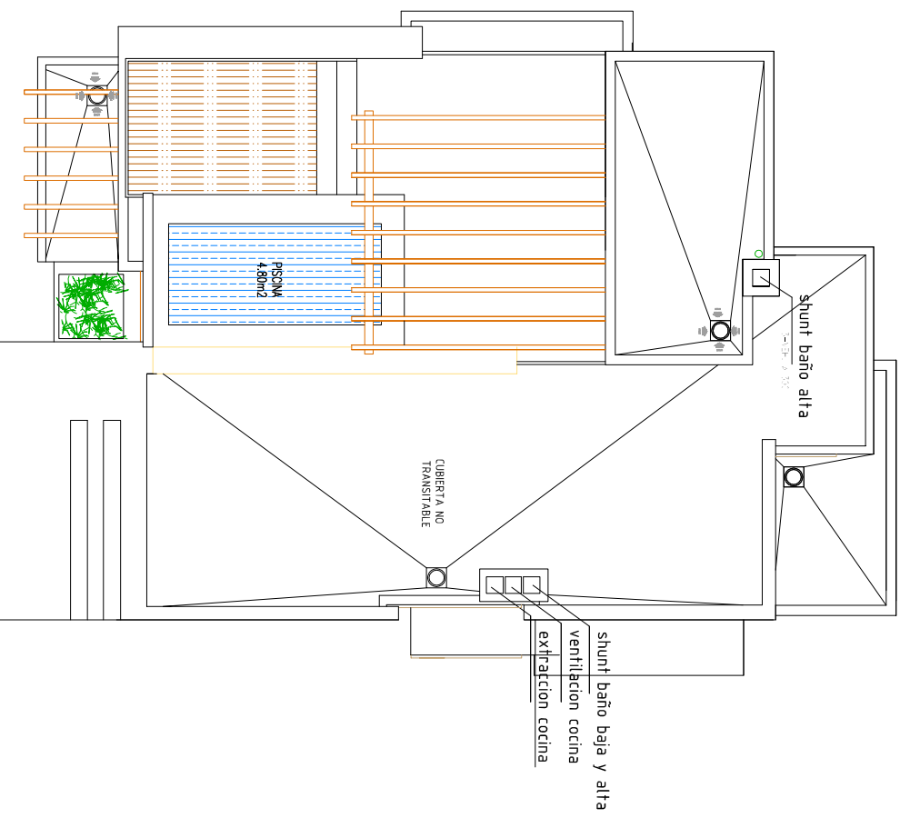
PLANTA CUBIERTAS
