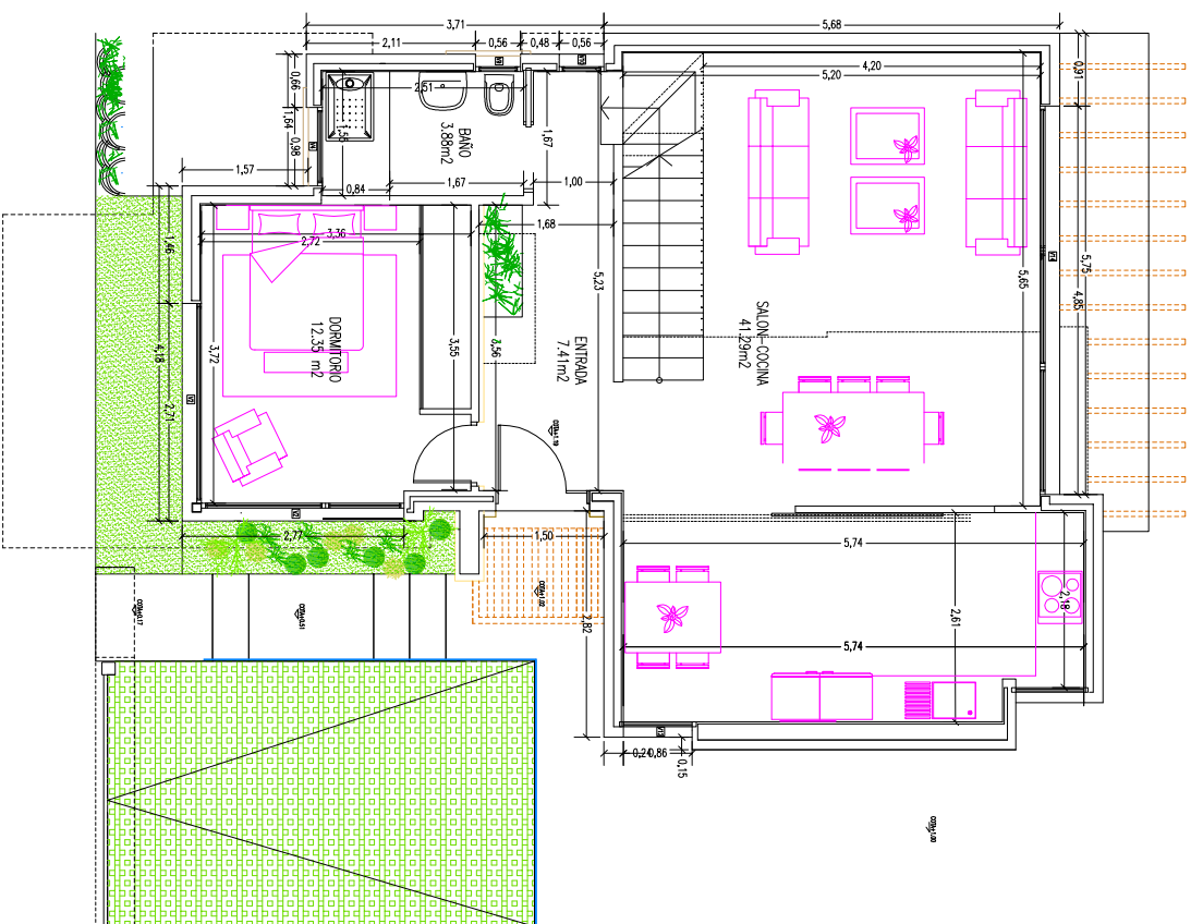
PLANTA BAJA
