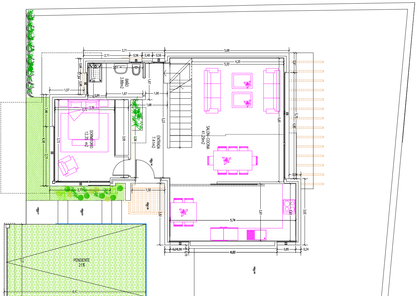
PLANTA BAJA
