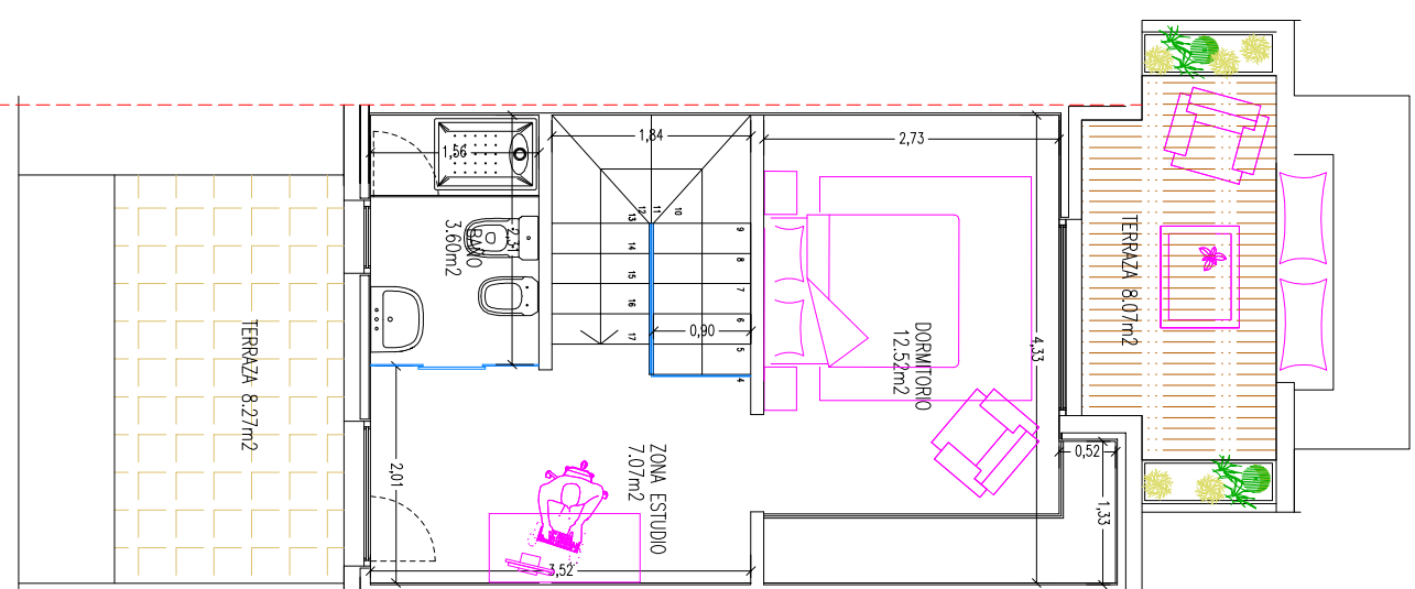
PLANTA ALTA
