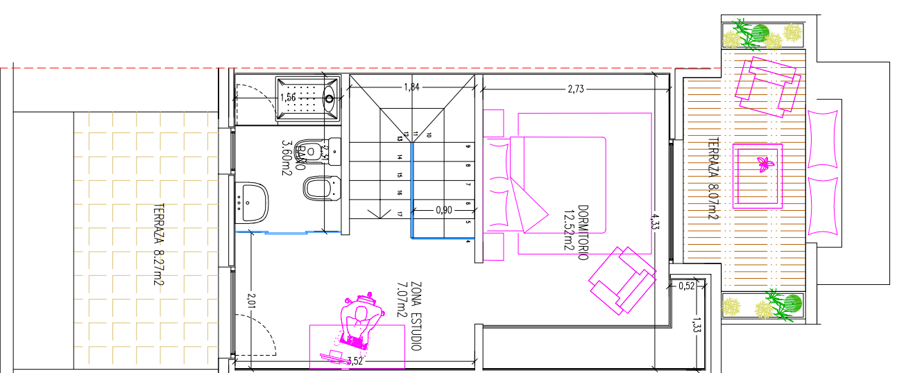
PLANTA ALTA
